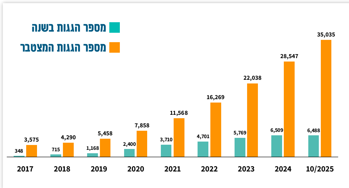
תרשים 6א': התקנות של מערכות קטנות, 2017-2025 (מעודכן לאוקטובר 2025)
