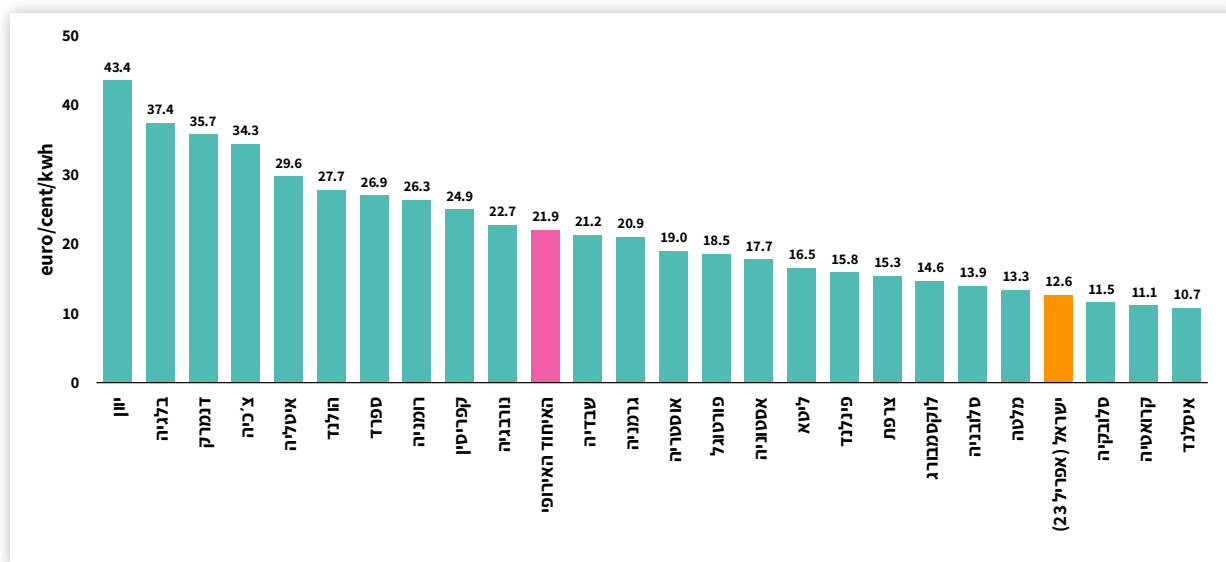
תרשים ב'2: השוואת מחיר החשמל בישראל לאיחוד האירופי (המקור: דו"ח ייצור החשמל בישראל, רשות החשמל, 2023)
