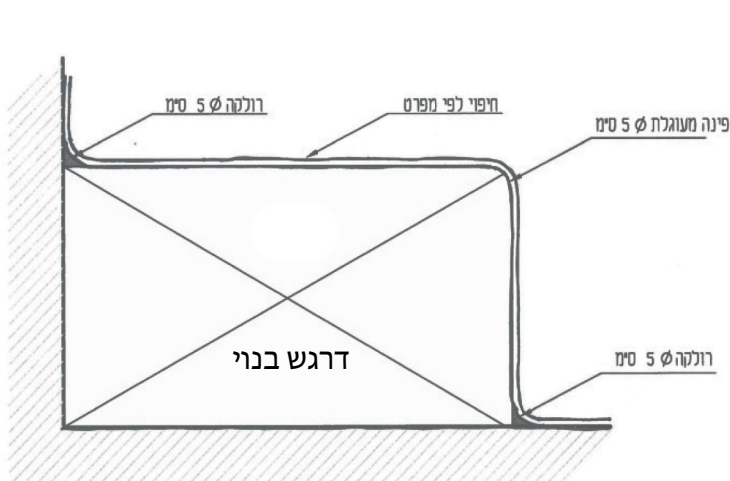
חתך 2-2
