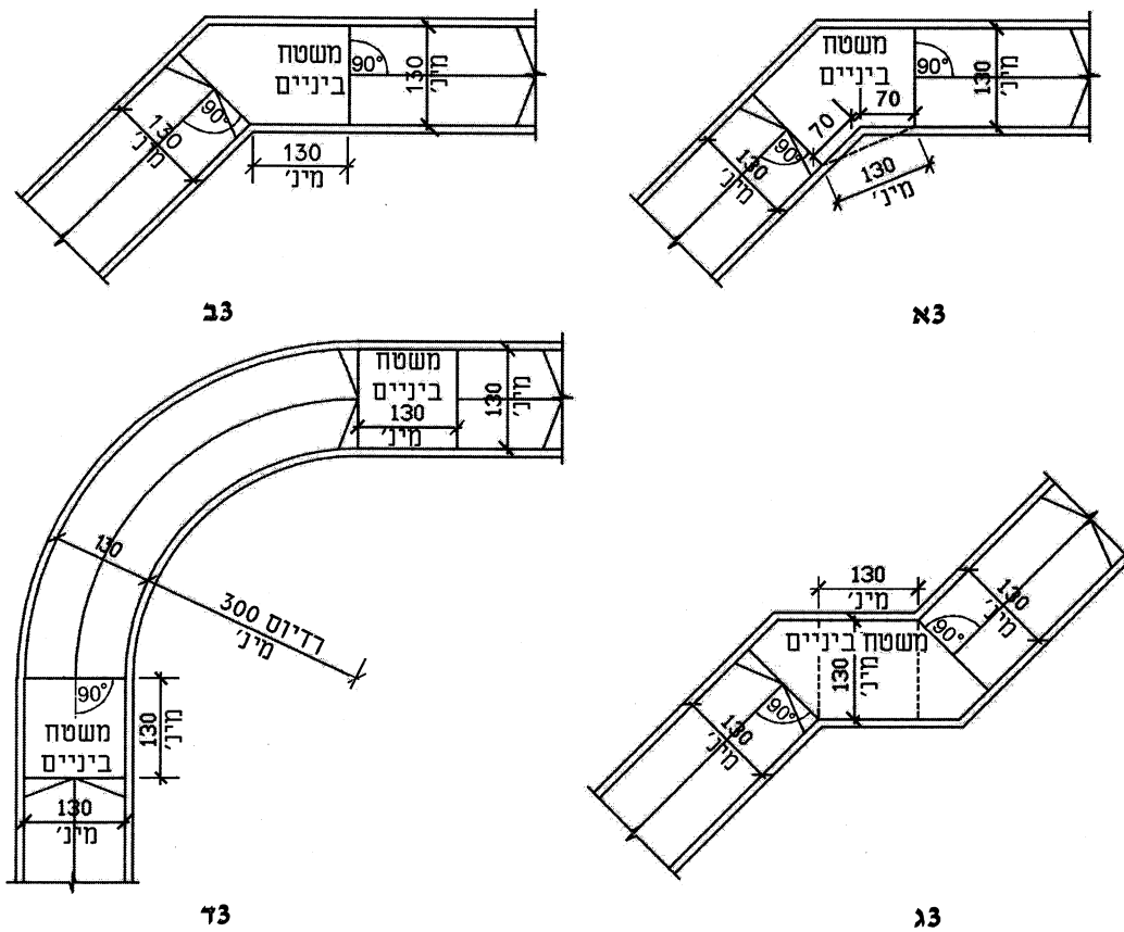
צור 3 – דוגמות למפגש בין כבש למשטח ביניים (המידות בסנטימטרים)
