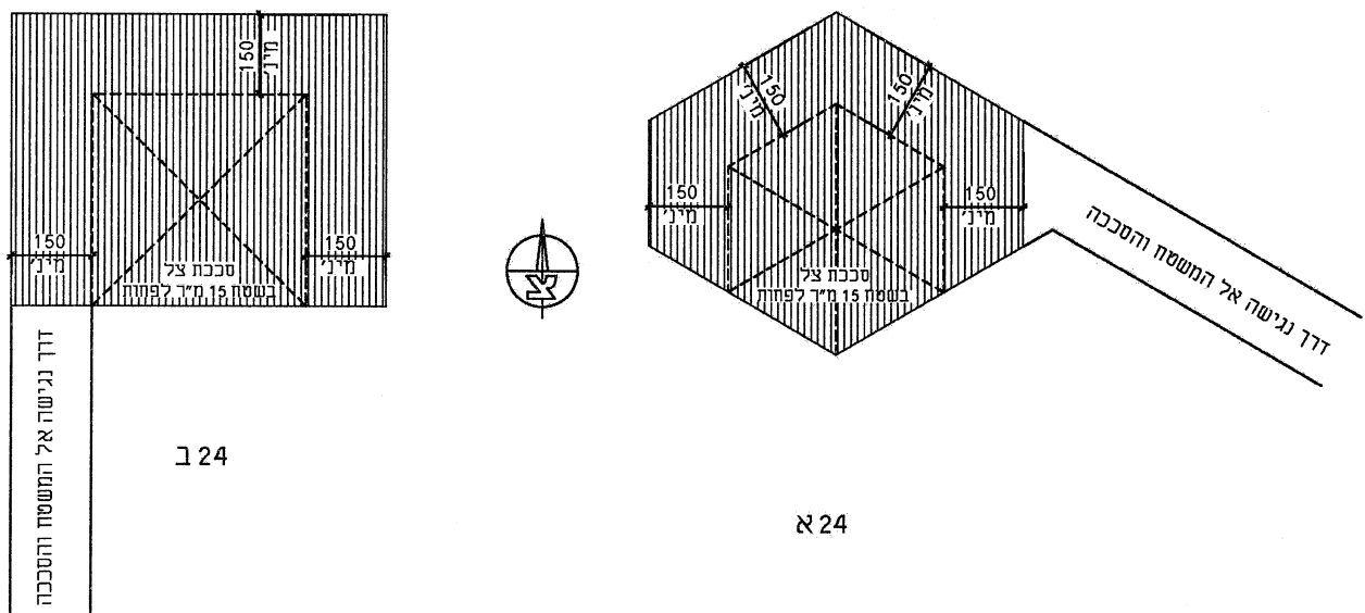
צור 25 – דוגמות לסככות צל נגישות (המידות בסנטימטרים)
