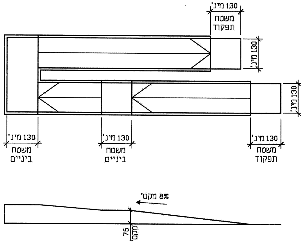
צור 2 – משטחי ביניים בכבש (המידות בסנטימטרים)
