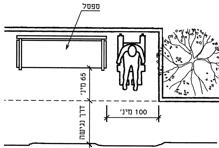
221 - ספסל - מבט על
