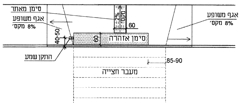
ציור 13 – דוגמה להנמכה במדרכה צרה (המידות בסנטימטרים)
