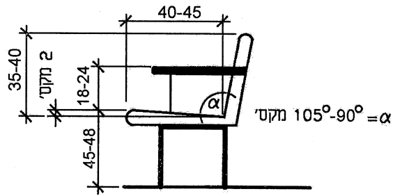
221 - ספסל - מבט צד
